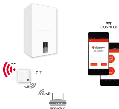
Δέκτης RF/Wi-Fi
