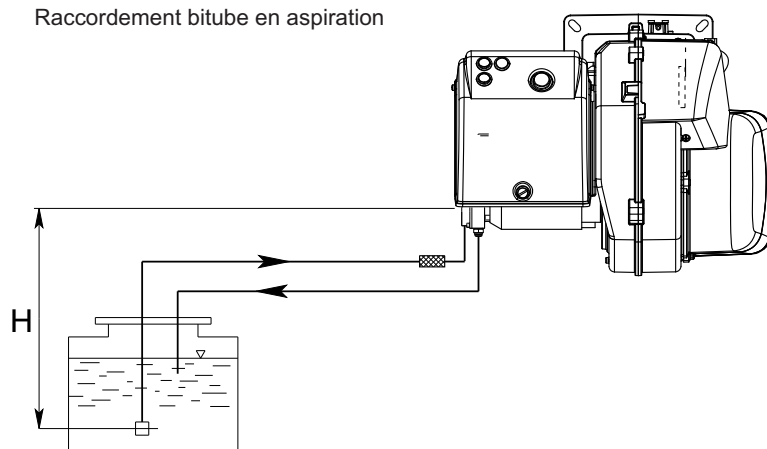
Raccordement bitube en aspiration
